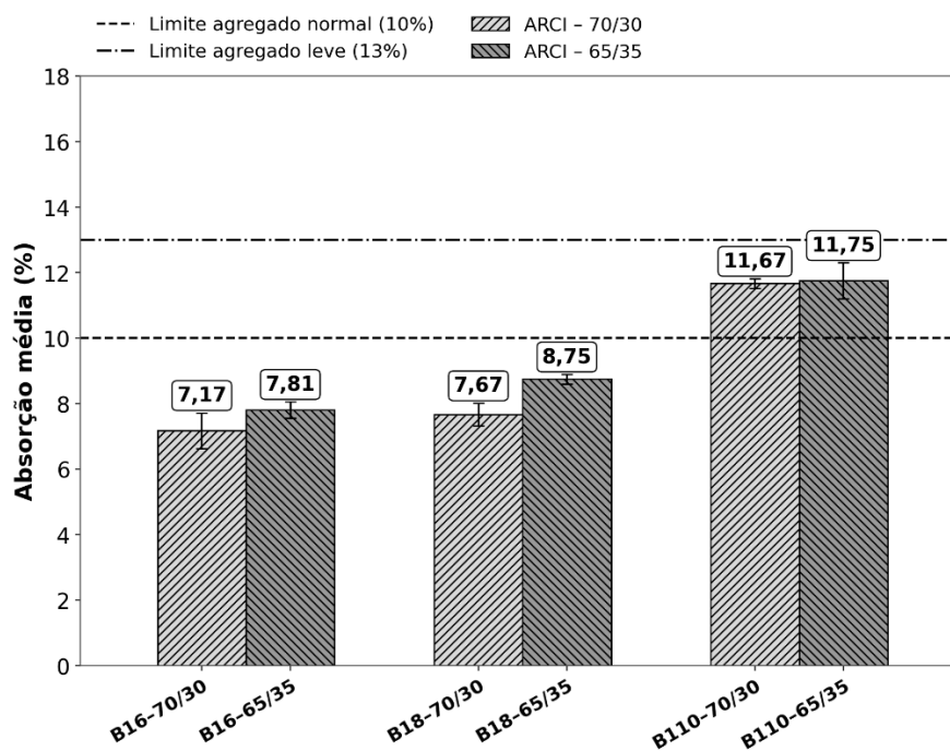
Figura 10. Absorção de água dos blocos de concreto com ARCI.
