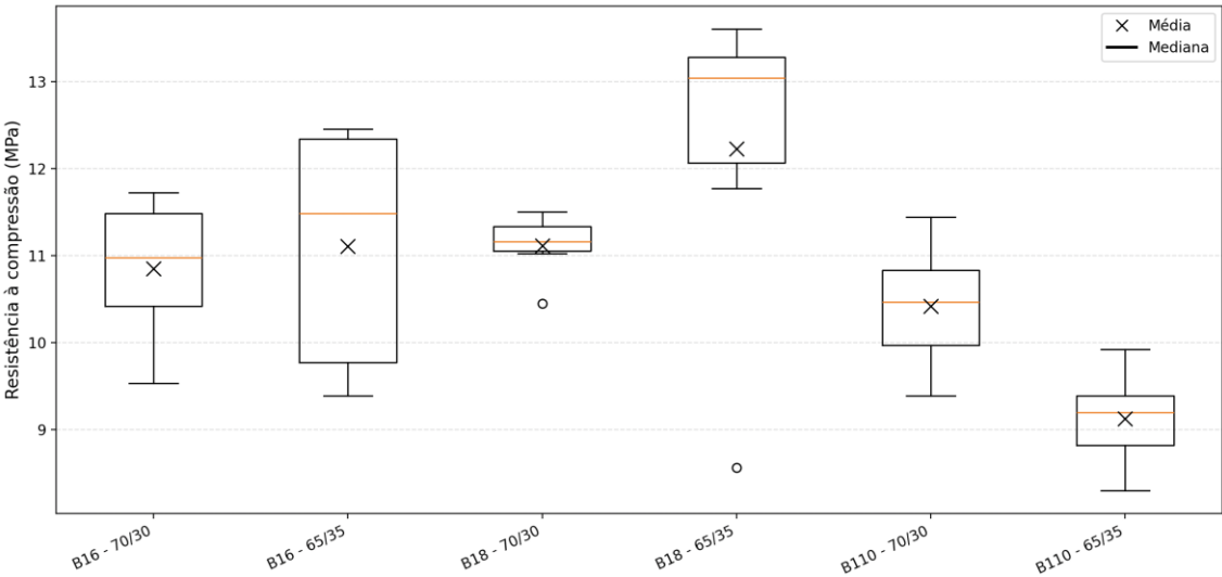
Figura 12. Boxplot dos experimentos: resistência à compressão aos 28 dias.
