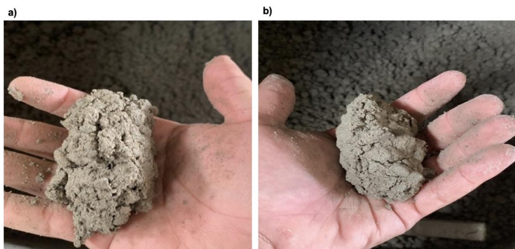
Figura 4. Aspecto do concreto com umidade de 7% e composições de agregados (%miúdo/%gráudo): (a) 65/35 e (b) 70/30.
