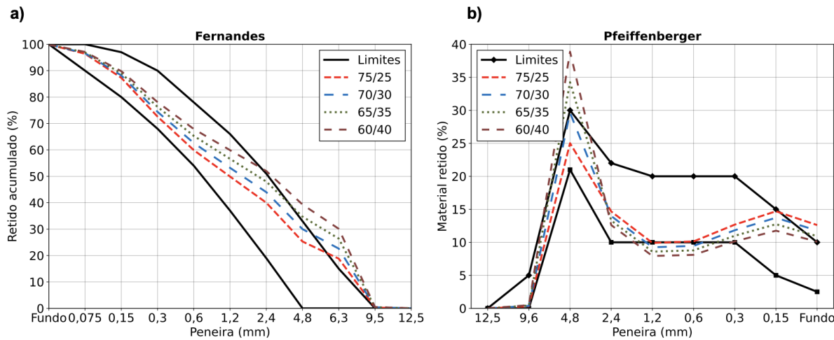
Figura 8. Curvas das composições de AMRCI e AGRCI: (a) Fernandes (2013) e (b) Pfeiffenberger (1985).
