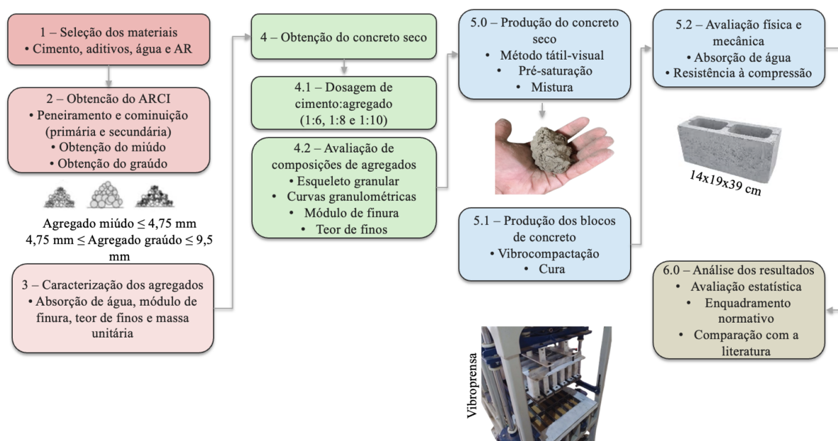
Figura 1. Fluxograma do delineamento experimental adotado no estudo.
