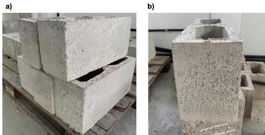
Figura 9. Aspecto visual dos blocos: (a) vista comprimento e (b) vista largura.
