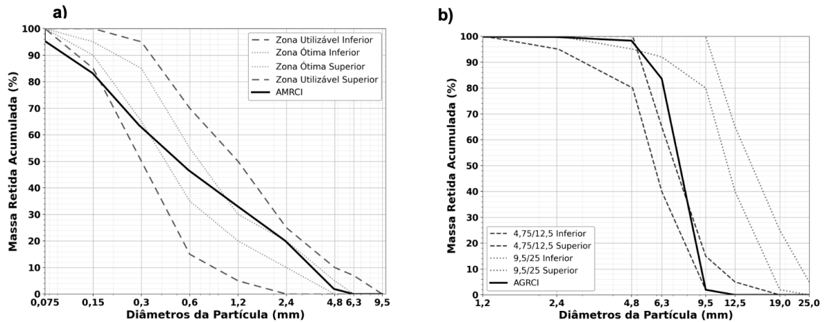
Figura 3. Composição granulométrica: (a) AMRCI e (b) AGRCI.
