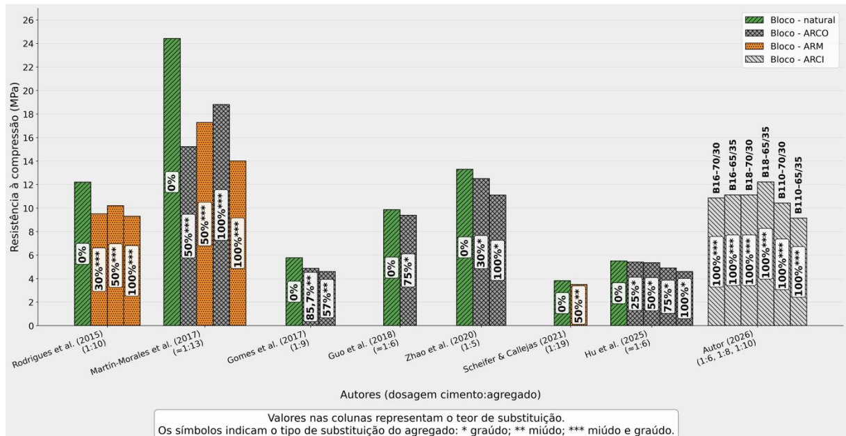
Figura 13. Resistência à compressão simples de blocos vazados de concreto seco.
