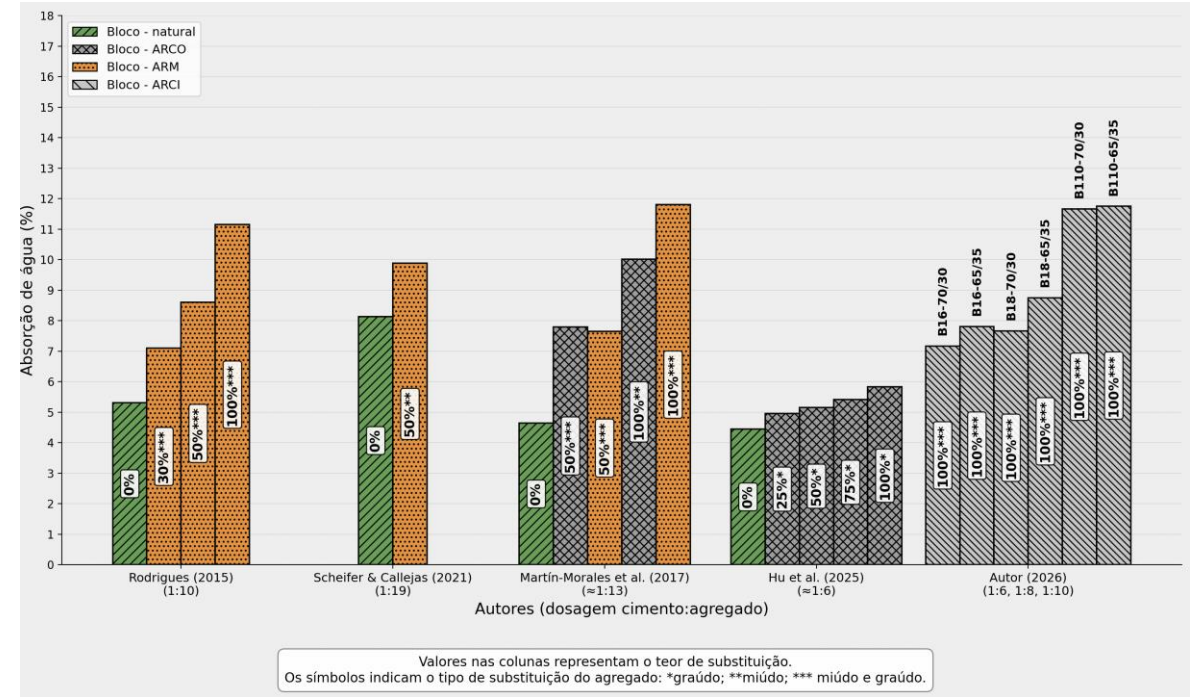
Figura 11. Absorção de água de blocos vazados de concreto seco.
