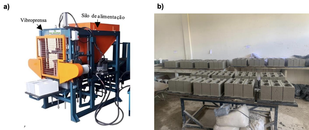
Figura 6. Em (a) Vibroprensa hidráulica e em (b) blocos recém produzidos.
