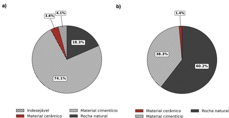
Figura 2. Composição dos constituintes do AGRCI: (a) material primário (MP) e (b) material secundário (MS).
