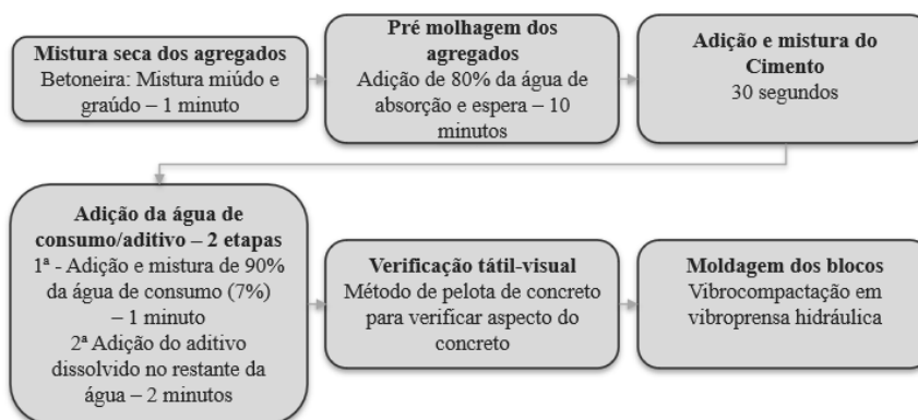
Figura 5. Fluxograma de produção do concreto seco.
