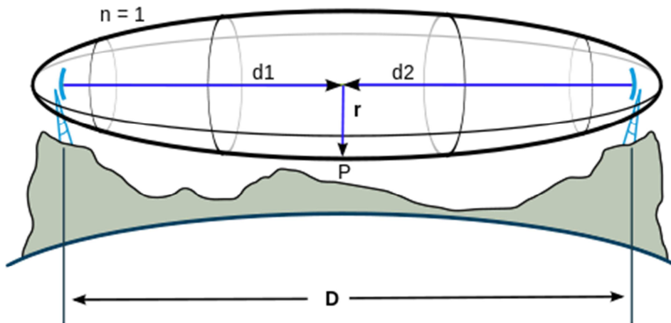
Figura 11 – Elipsóide de Fresnel Fonte – (MEHL, 2011)
