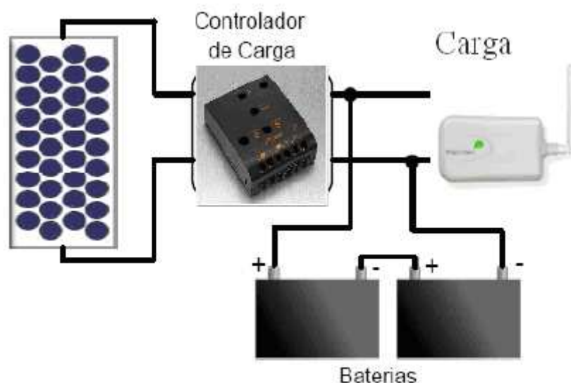
Figura 10 – Sistema montado através de diagrama em blocos
