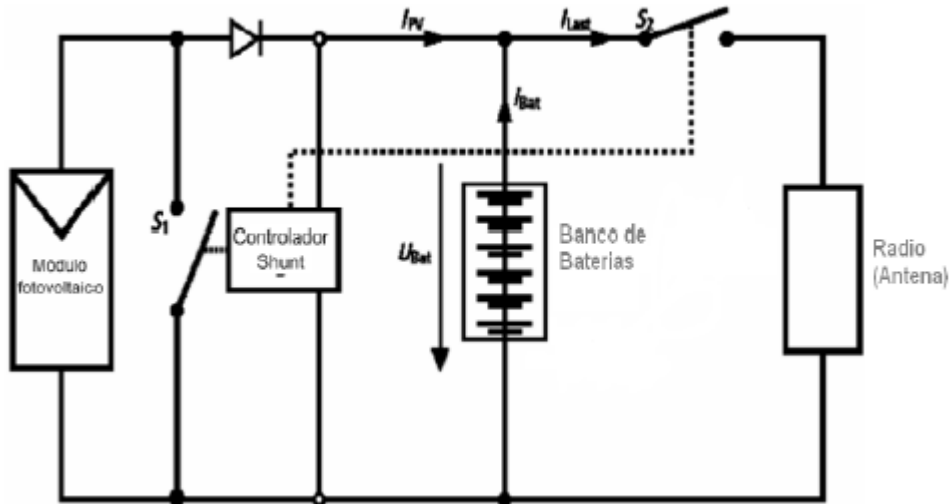
Figura 8 – Controlador de carga paralelo (shunt) (on/off)
