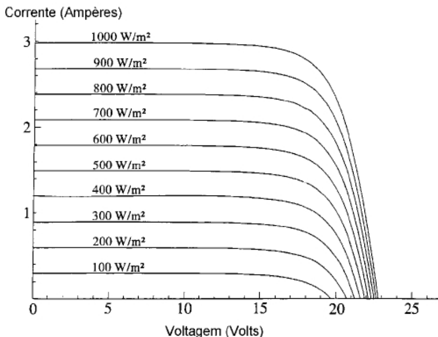
Figura 5 – Efeito causado pela variação de intensidade luminosa.
