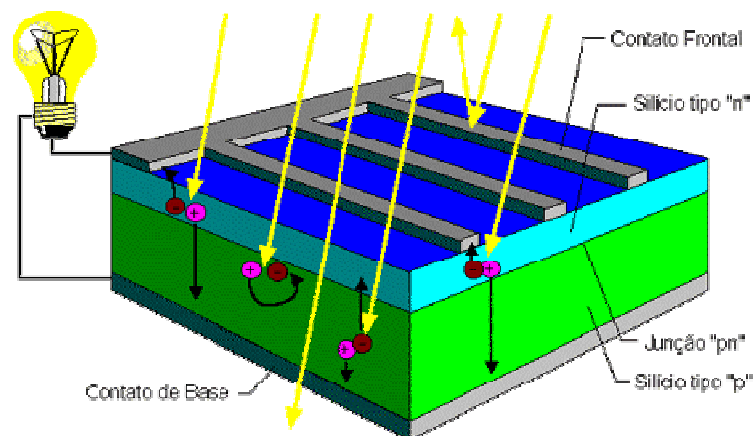
Figura 4 – Como funciona uma célula fotovoltaica
