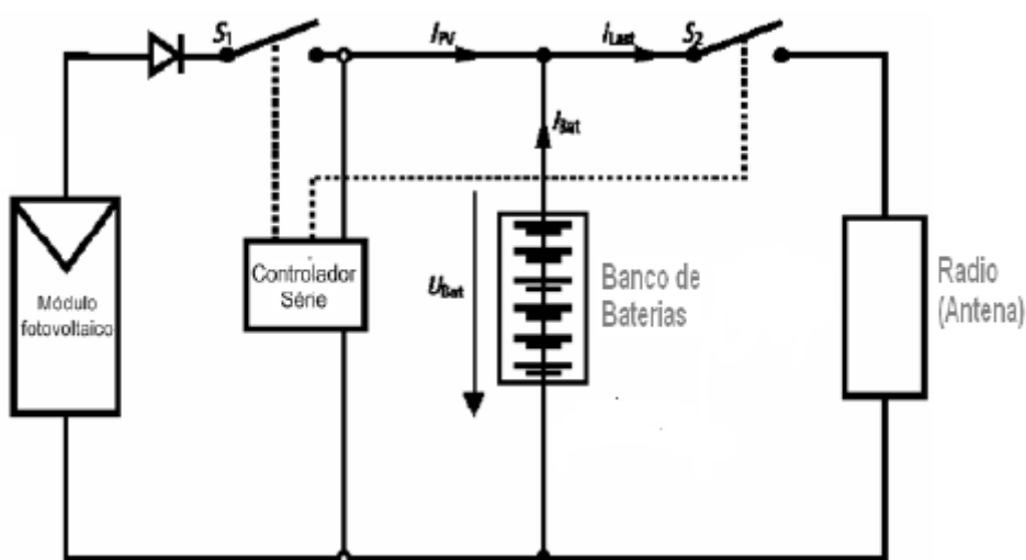
Figura 7 – Controlador de carga serie (on/off) –
