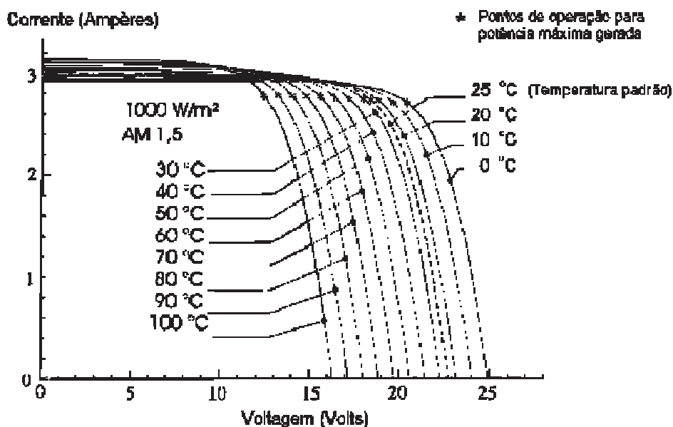
Figura 6 - Efeito causado pela temperatura na célula.
